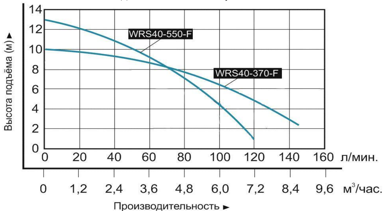
5.14. Модель WRS40-370-F, WRS40-550-F.
