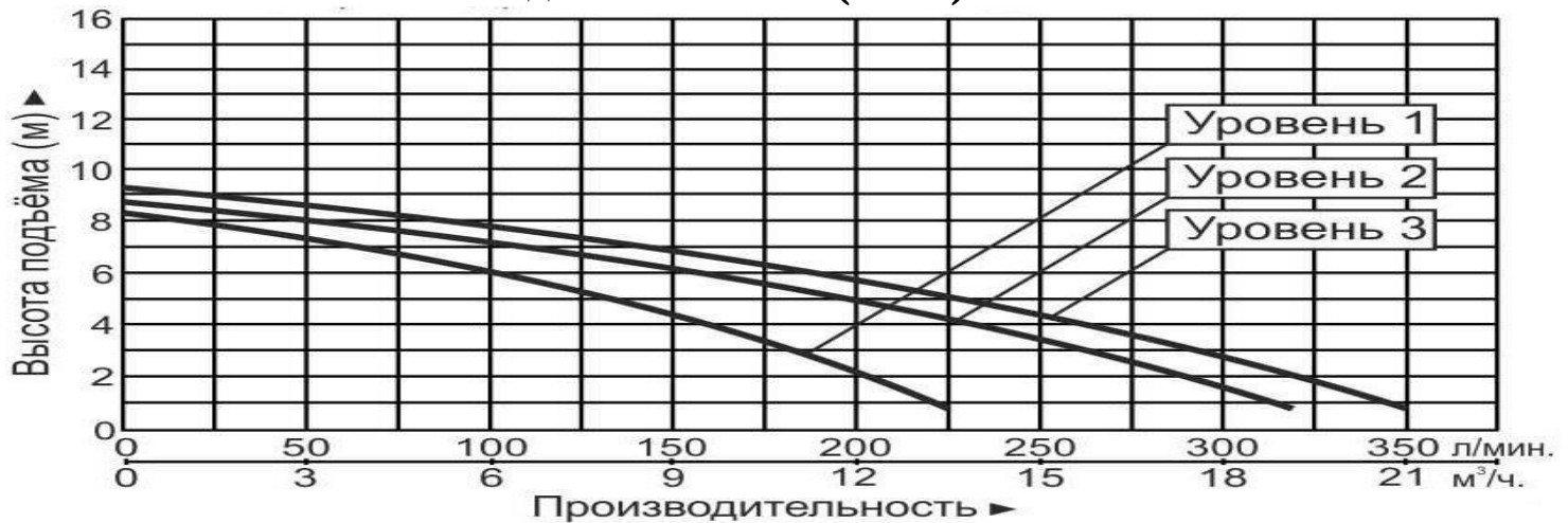
5.18. Модель GRS50-9F(380V)-Premium.
