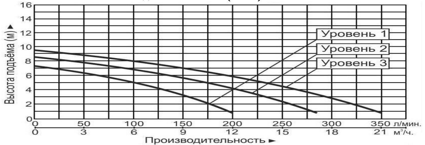
5.19. Модель GRS50-13F(220V)-Premium.
