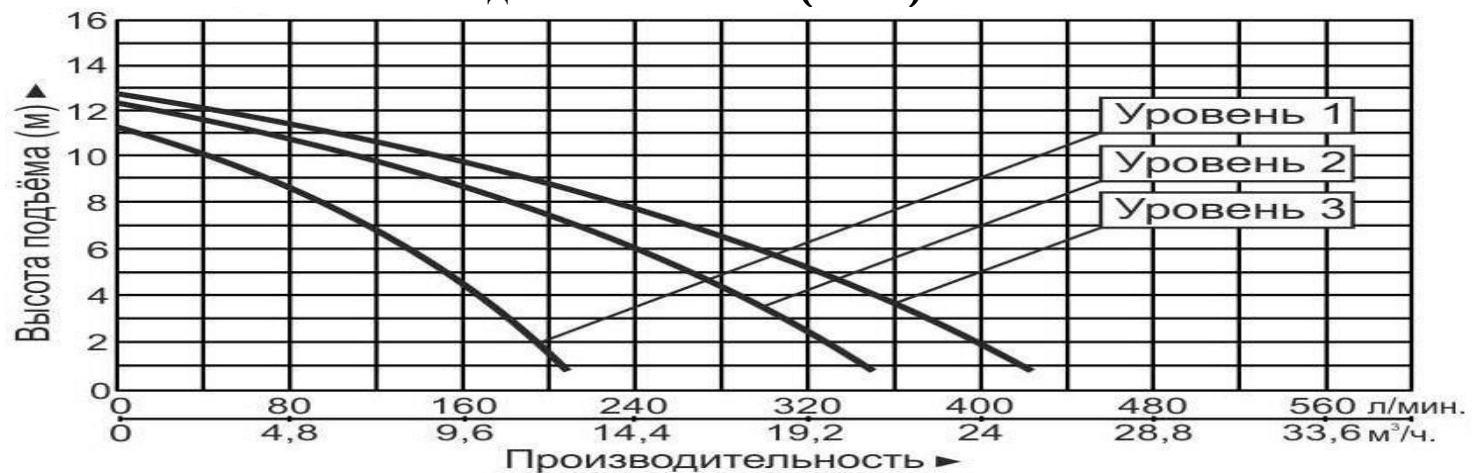
5.19. Модель GRS50-13F(220V)-Premium.
