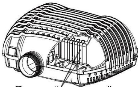
Датчики «сухого хода»
