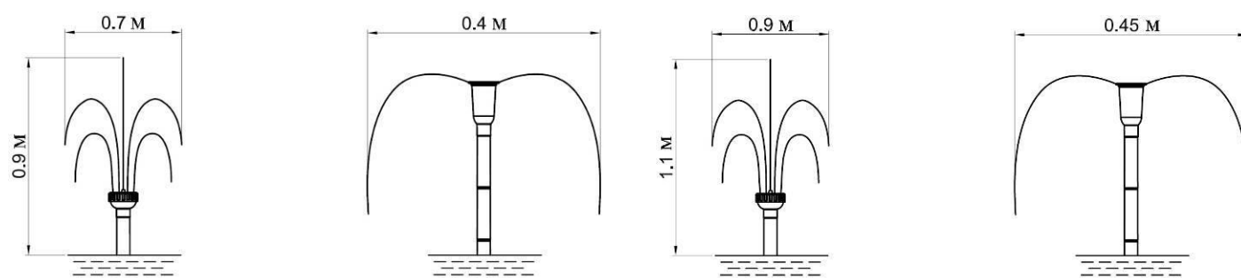
Для модели НФСП-350л/ч-0,9м
