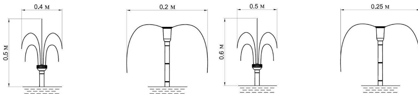
Для модели НФСП-240л/ч-0,5м
