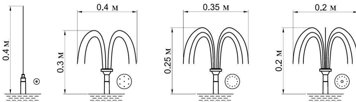
Для модели НФСП-70л/ч-0,5м
