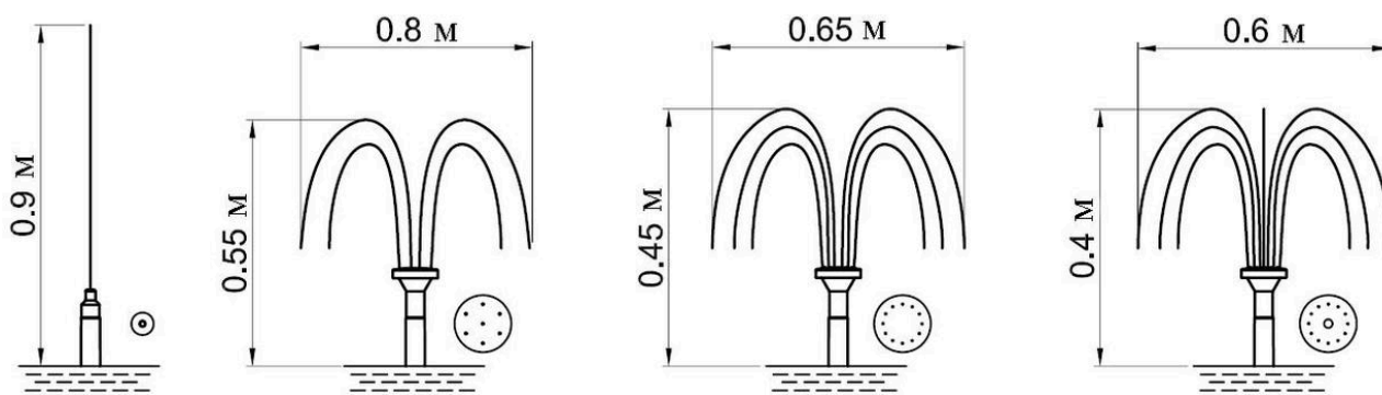
Для модели НФСП-160л/ч-0,6м
