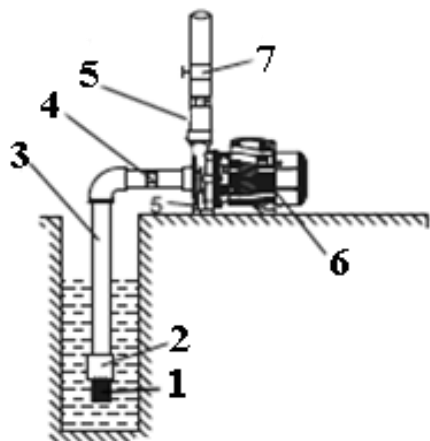
Правильная установка.
