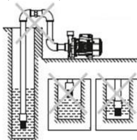
Неправильная установка.
