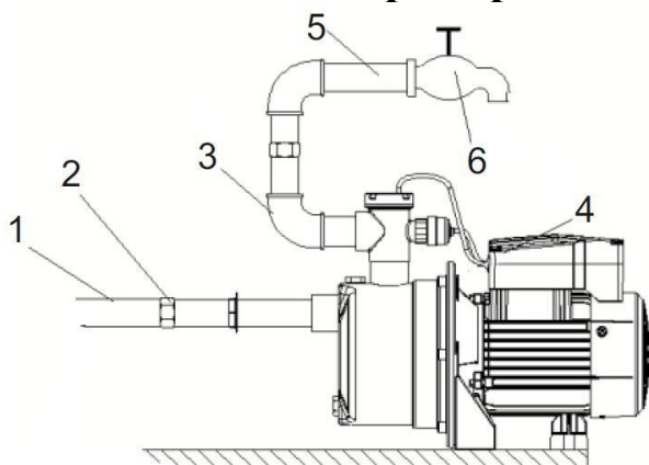
Правильная установка насоса.
