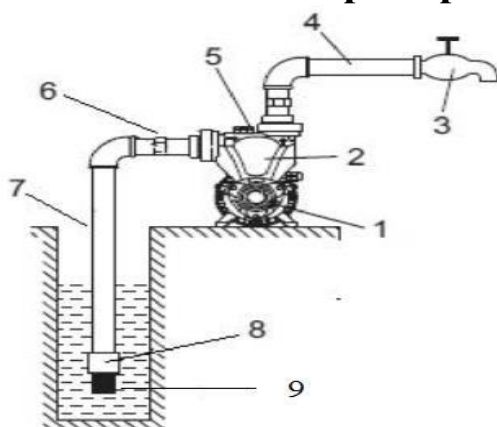
Правильная установка.
