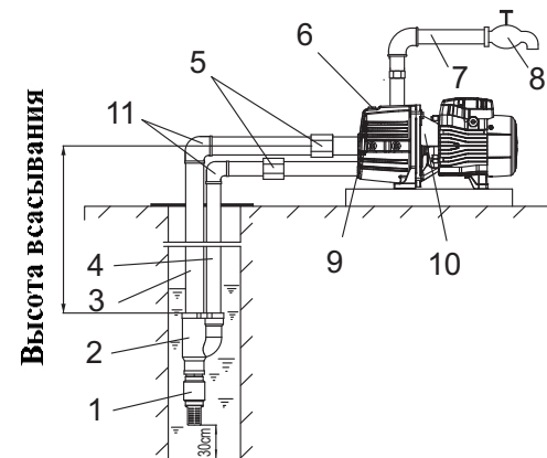
Рис. 7. Схема установки насосов моделей AJDm55/4H, AJDm75/4H, AJDm110/4H.
