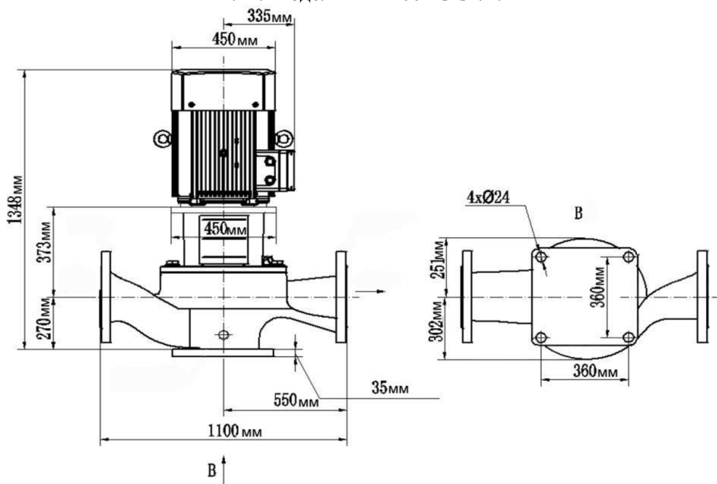
7.24. Модель LPP200-23-37/4.
